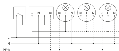
Diagrama electrónico lámpara con conductor neutro
